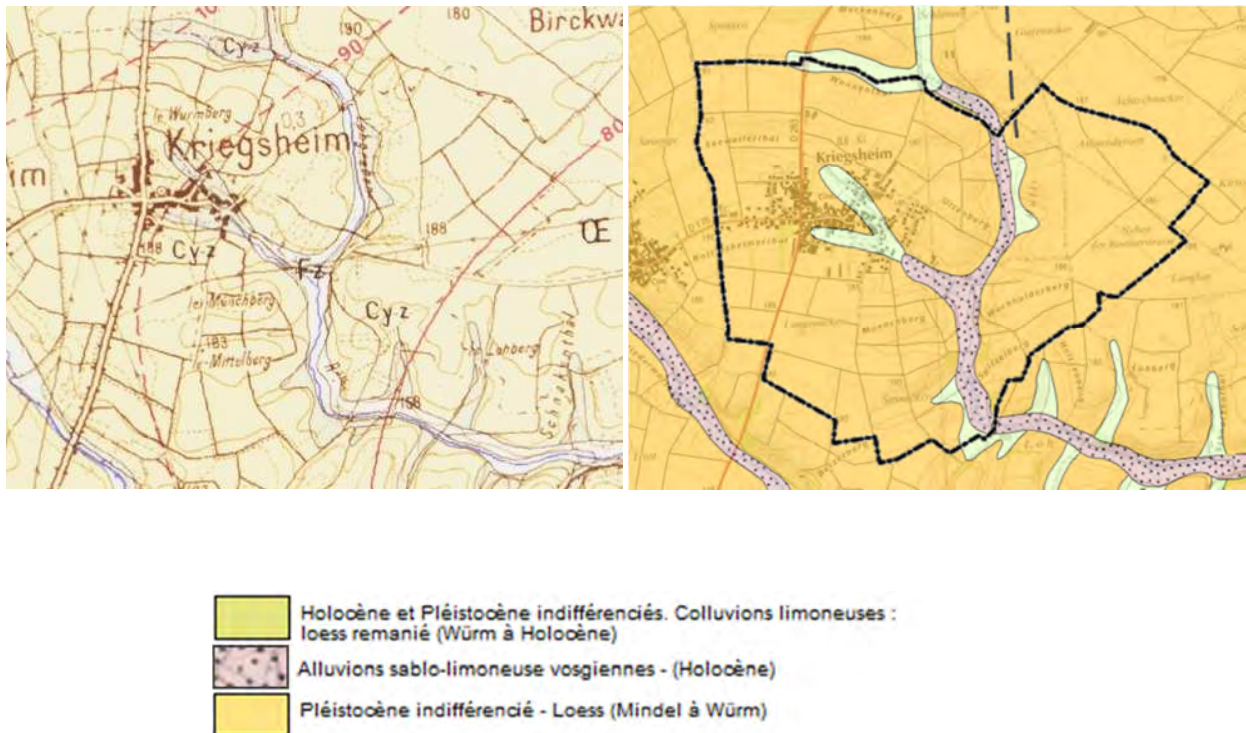
Carte géologique du Kriegsheim (source : BRGM)
